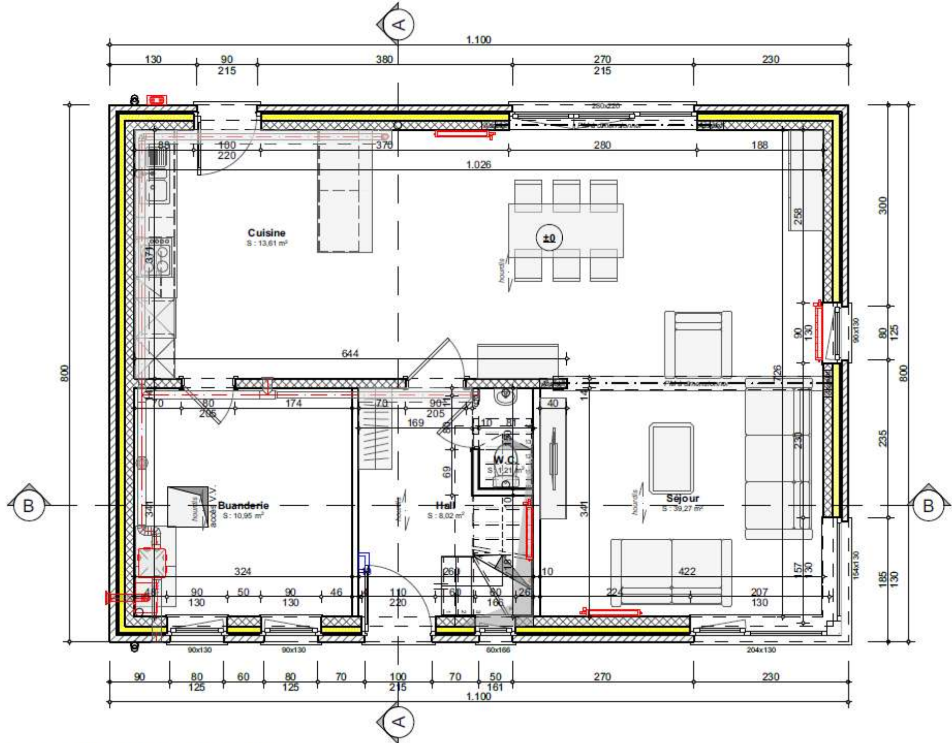
Rez-de-chaussée
